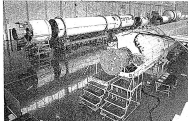
工場内に横たわるH1ロケット
